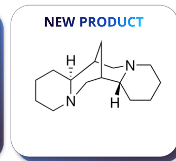
Sparteine
